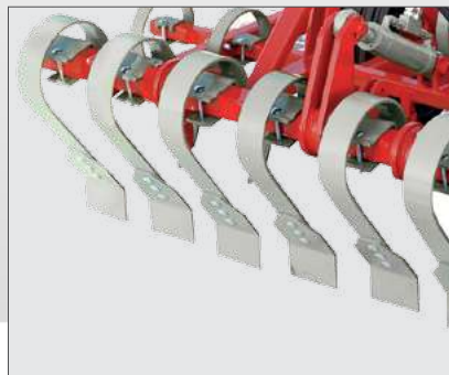
Передня пружинна волокуша з гідрорегулюванням (hydrokrossboard) гарантує якісне вирівнювання поля
