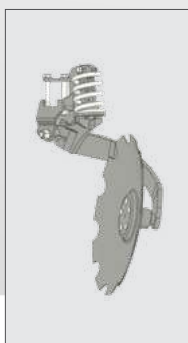
TX 660 Aggressive - один диск на стійці з пружинним захистом
